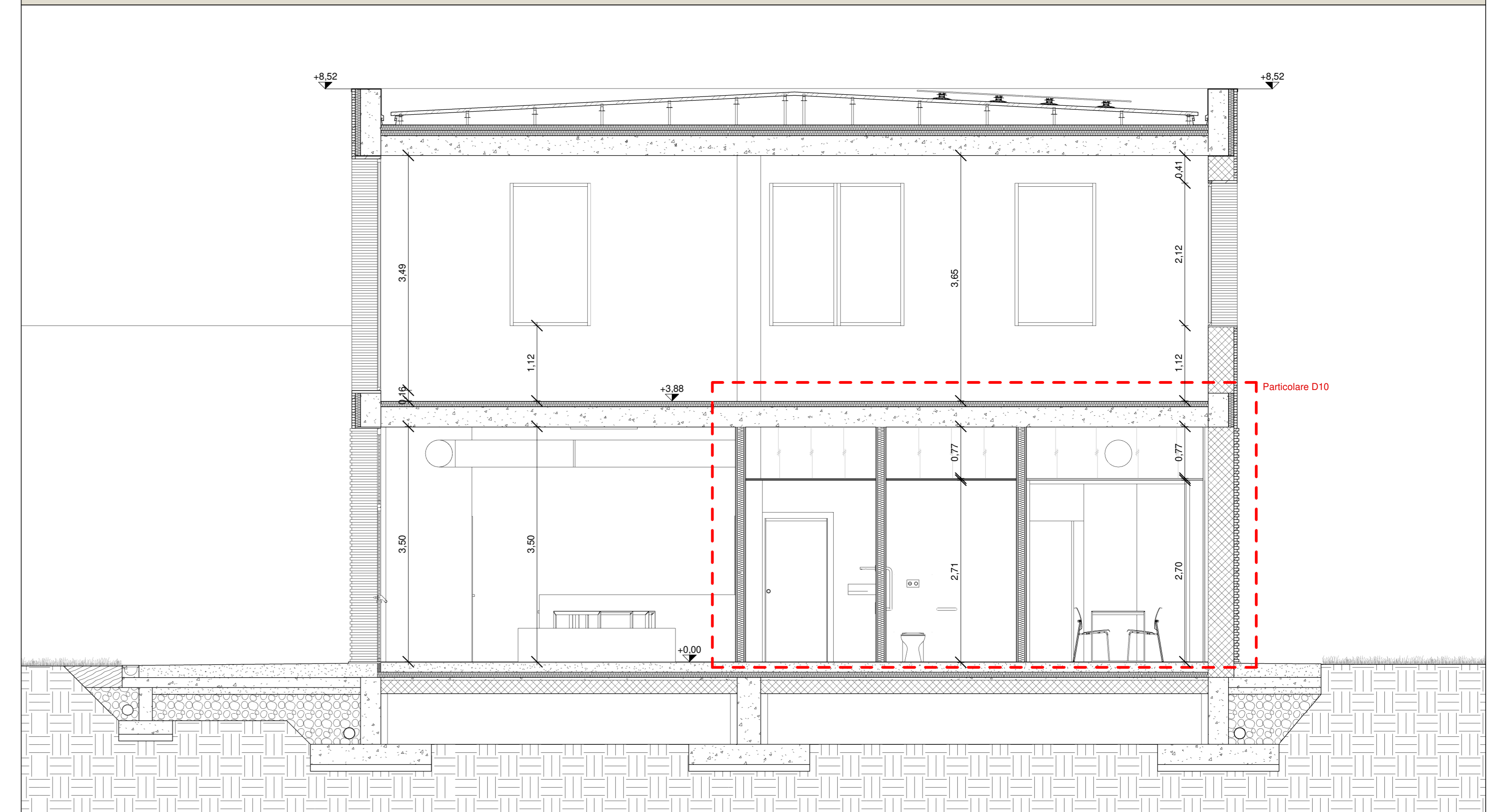
Sezione E-E' _SCALA 1:50
