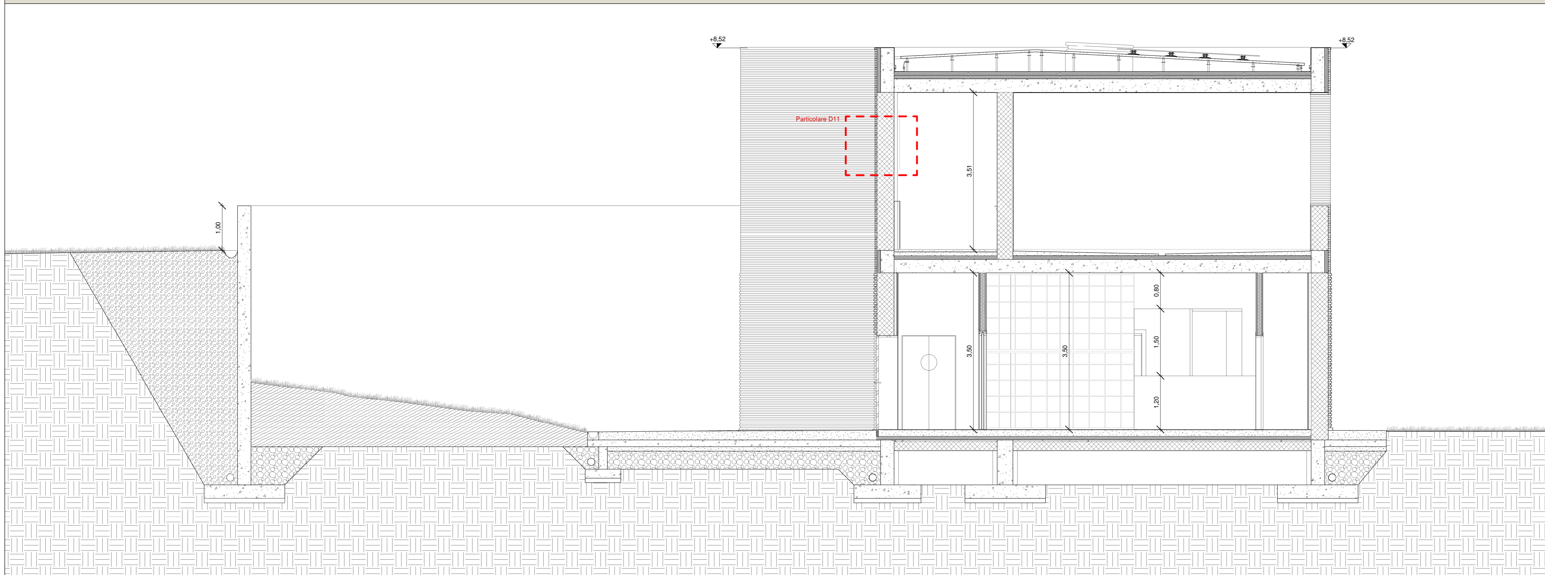
Sezione C-C' _SCALA 1:50
