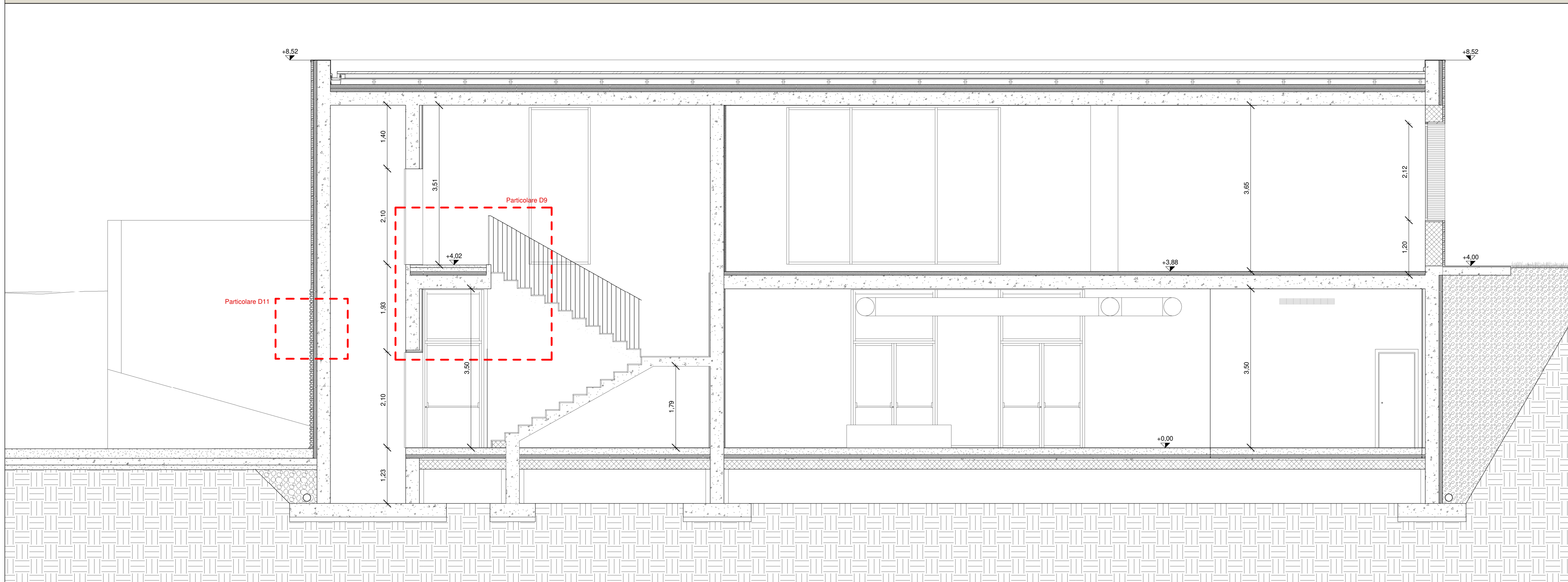
Sezione B-B' _SCALA 1:50
