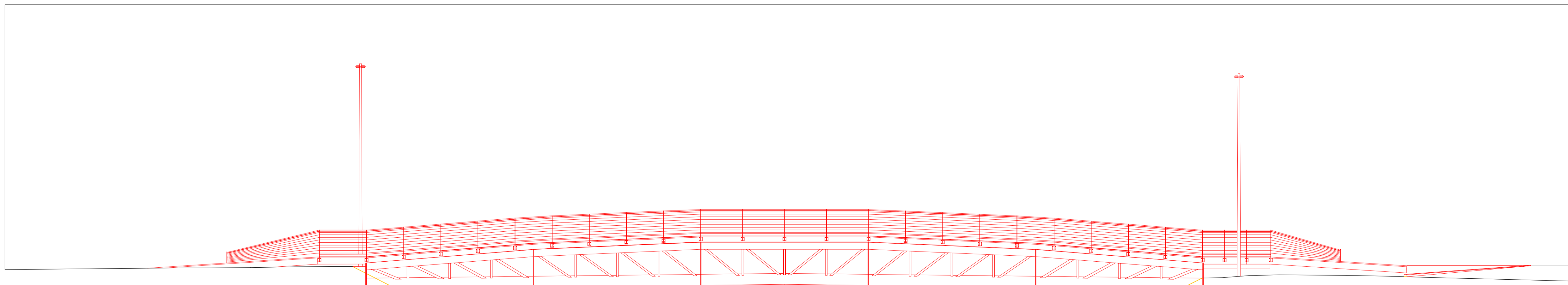
Sezione a - a vista da sud - stato sovrapposto scala 1:100
